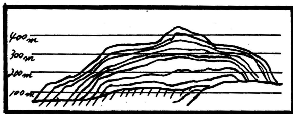
昭和新山 (三松ダイヤグラム) 三松先生が観測した山の成長図です。 1947年オスローの万国火山会議に提出し、賞讃された原図を写したものです。
